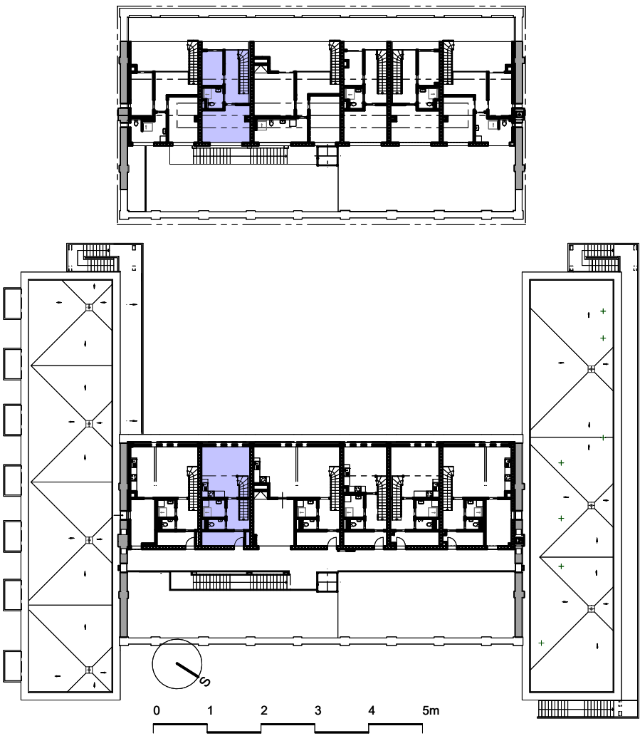
Schéma půdorys
